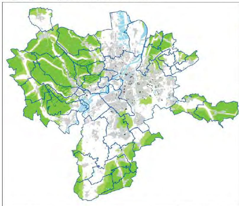
Cartographie des zones pour lesquelles le niveau sonore multiexposé en Lden est inférieur à 55 dB(A) croisé avec zones Natura2000
