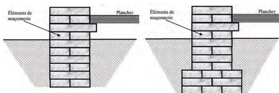
Figure 8 Fondation en maçonnerie (semelle filante ou isolée)
