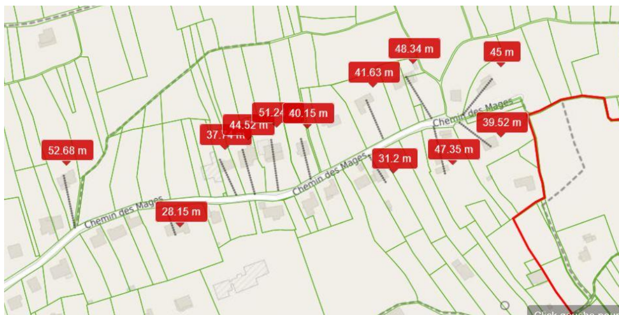
Implantation du bâti existant par rapport au domaine public – Zone des Coteaux (Chemin des Mages)
